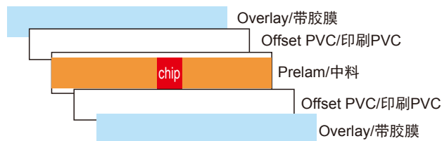
结构图(Structure)
