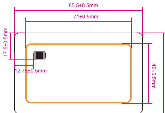
天线 (Antenna)
